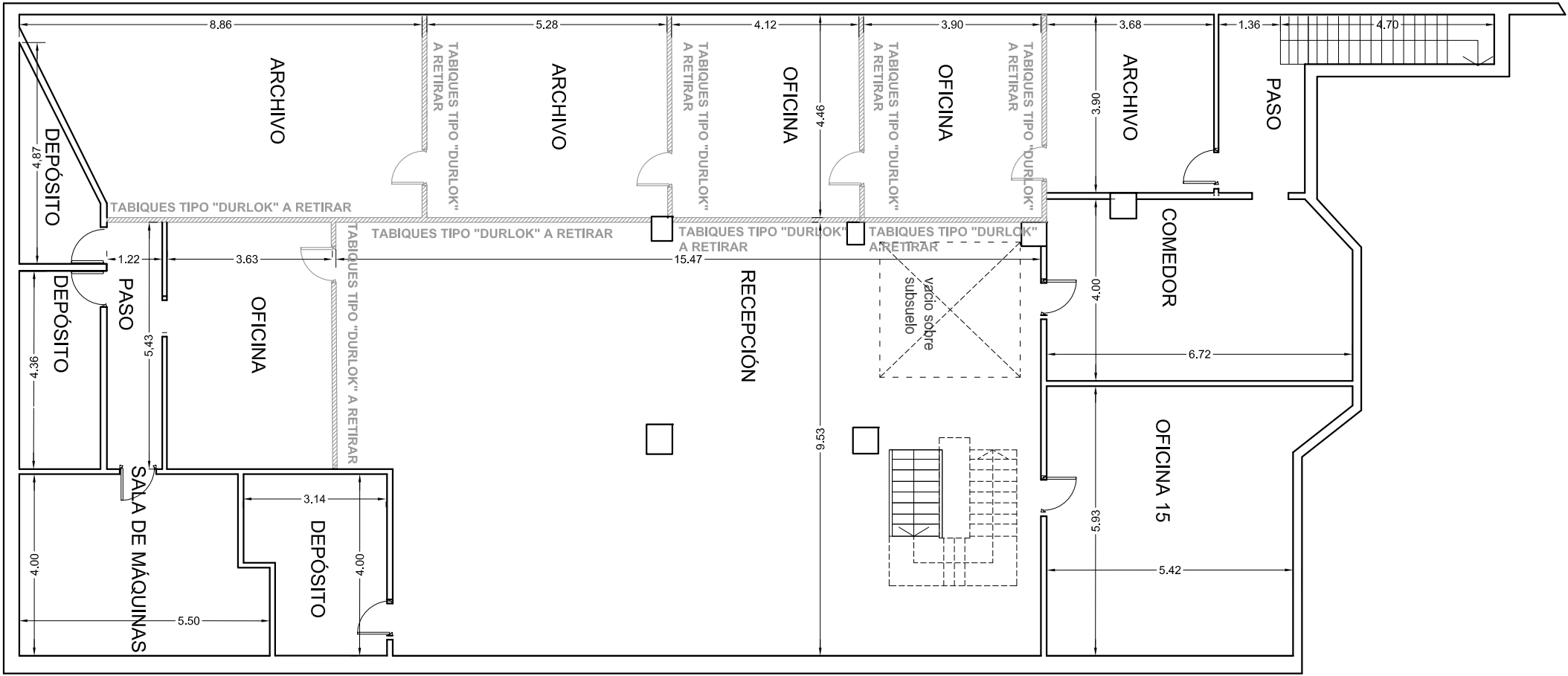
PLANTA SUBSUELO
